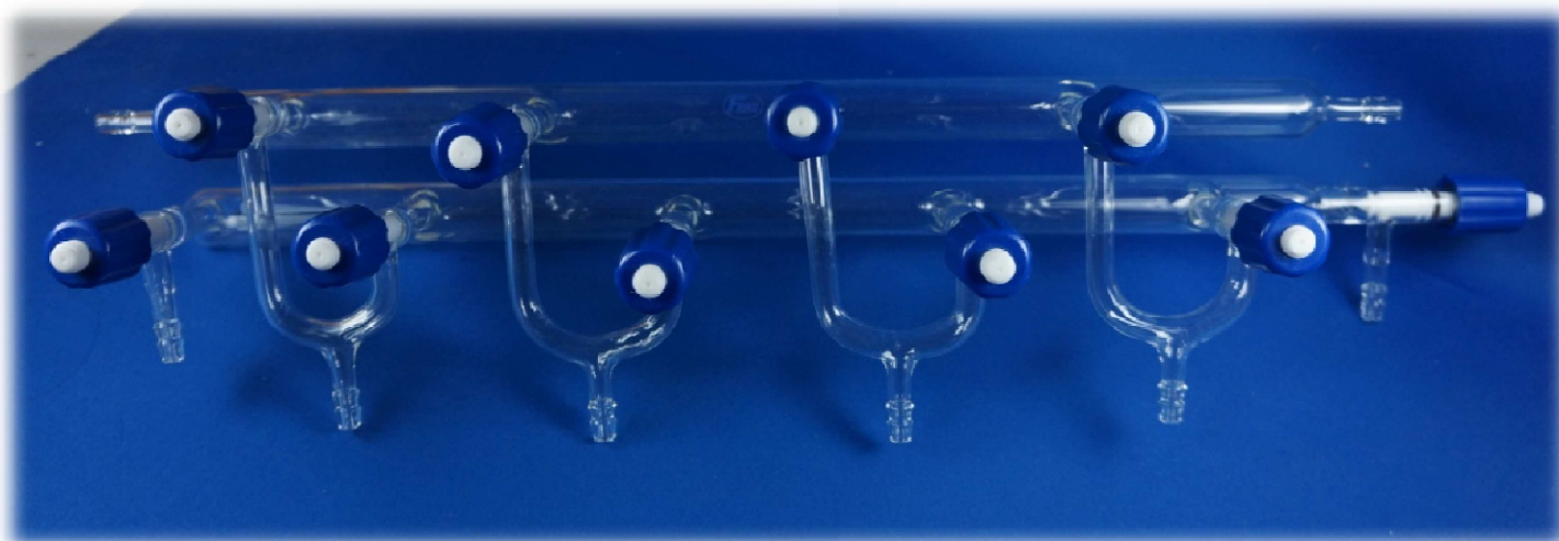
ガス置換真空マニフォールド バルブ使用
