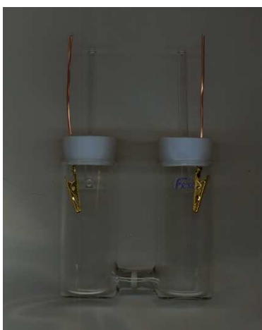
2連電解セル フィルター&amp;Cu電極付
