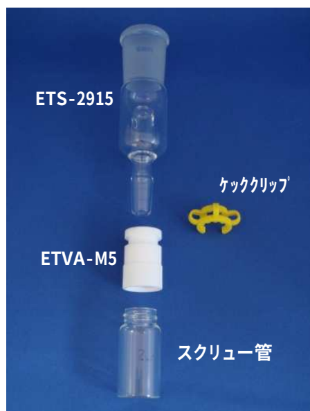
スクリュー管とバイアル瓶アダプターと専用トラップ管の接続
